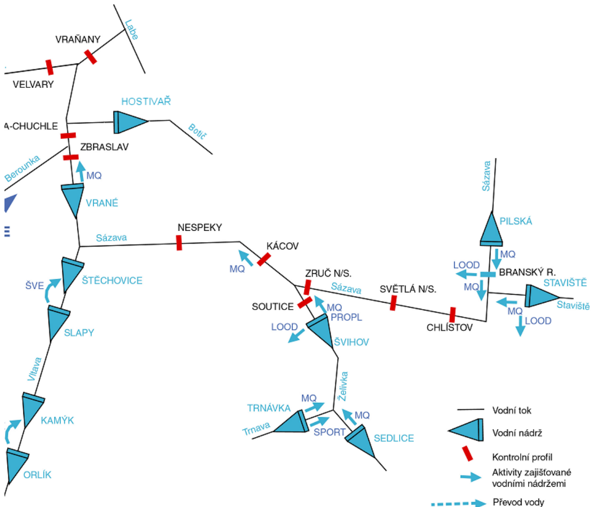
Obr. 2.4.1 Základní struktura vodohospodářské soustavy v dílčím povodí Dolní Vltavy
