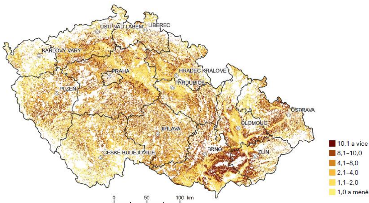
Obrázek II.1.1b Potenciální ohroženost zemědělské půdy vodní erozí vyjádřená dlouhodobým průměrným smyvem půdy v ČR ( t \cdot ha^{-1} \cdot rok^{-1} ) 2017 [14]
