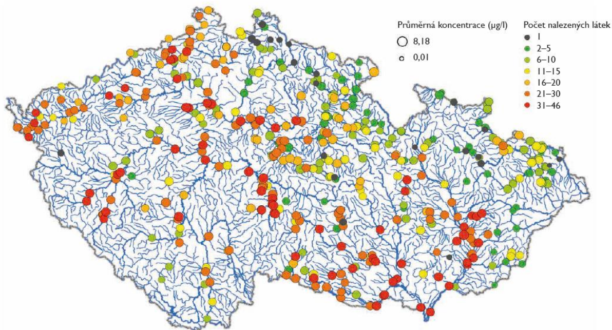
Obrázek II.1.1a Pesticidy na území České republiky dle počtu a koncentrace v roce 2018
