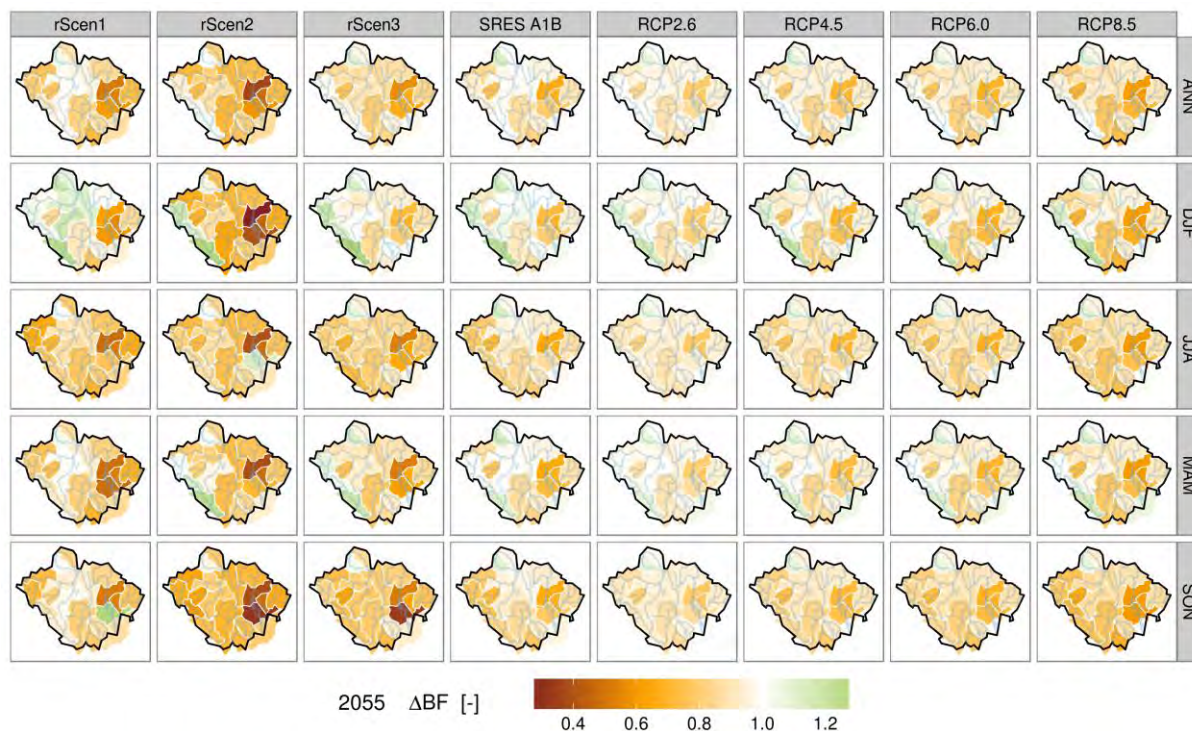
Obr. II.2.5b - Změna průměrných ročních výšek základního odtoku scénáře pro dílčí povodí Horní Vltavy a rok 2055
