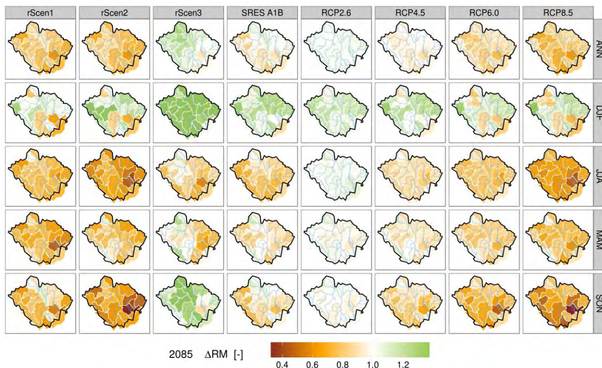
Obr. II.1.5i - Změna průměrných ročních odtokových výšek pro dílčí povodí Horní Vltavy a rok 2085
