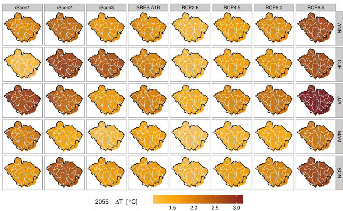
Obr. II.1.5e - Změna teploty pro dílčí povodí Horní Vltavy a rok 2055
