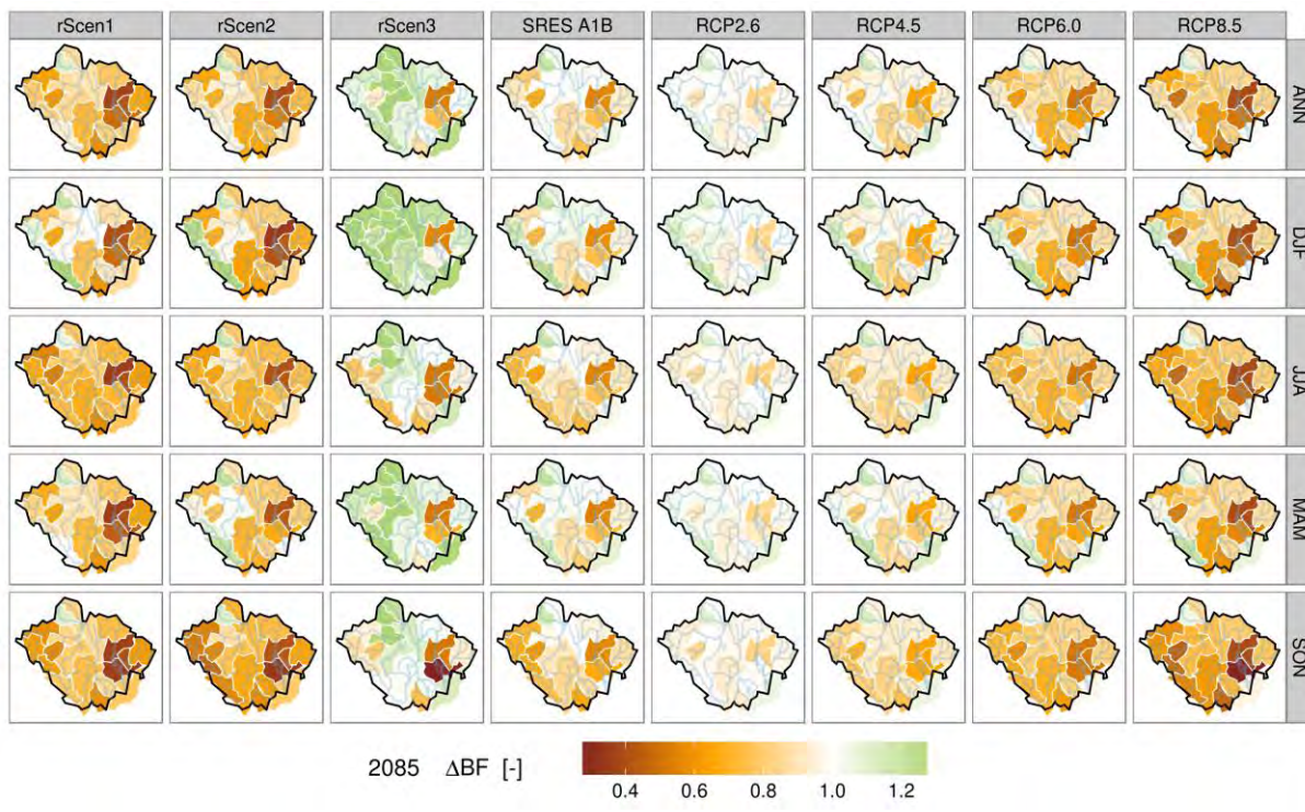
Obr. II.2.5c - Změna průměrných ročních výšek základního odtoku scénáře pro dílčí povodí Horní Vltavy a rok 2085
