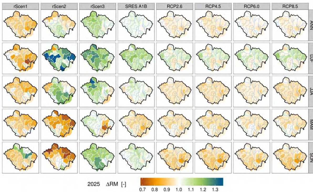
Obr. II.1.5g - Změna průměrných ročních odtokových výšek scénáře pro dílčí povodí Horní Vltavy a rok 2025
