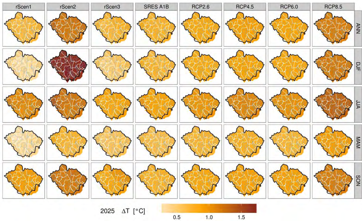
Obr. II.1.5d - Změna teploty pro dílčí povodí Horní Vltavy a rok 2025
