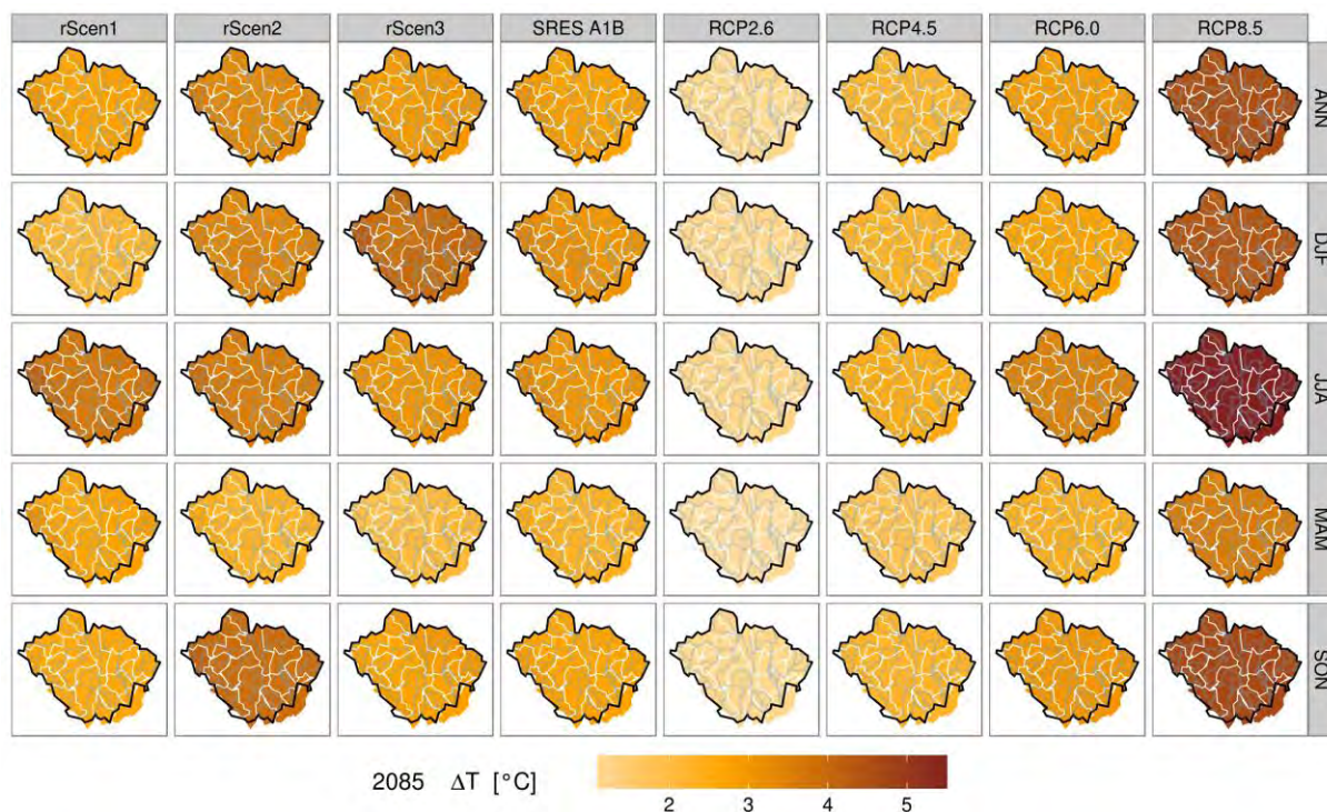
Obr. II.1.5f - Změna teploty pro dílčí povodí Horní Vltavy a rok 2085
