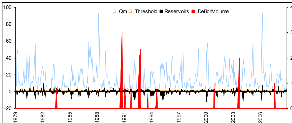
Obr. 7 Manipulace na kontrolním profilu Kácov (černě) a deficitní objemy (červeně) pro threshold Q95%
