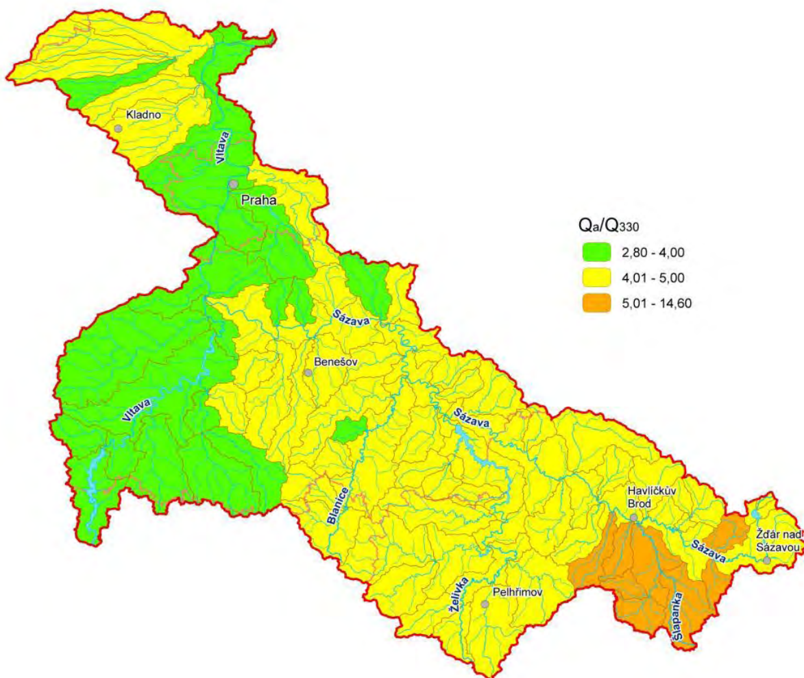
Obr.5 Poměr průtoků Q_a/Q_{330}
