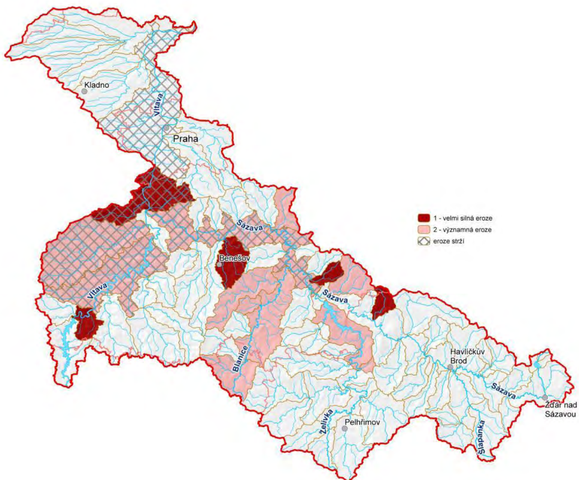
Obr.4 Vodní útvary ohrožené říční erozí
