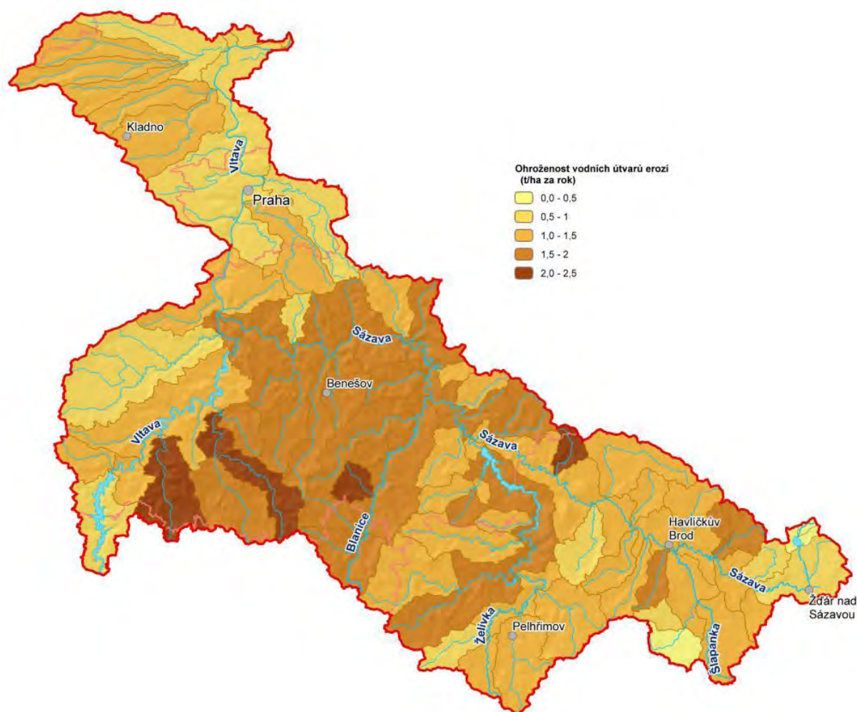
Obr.3. Plošná vodní eroze
