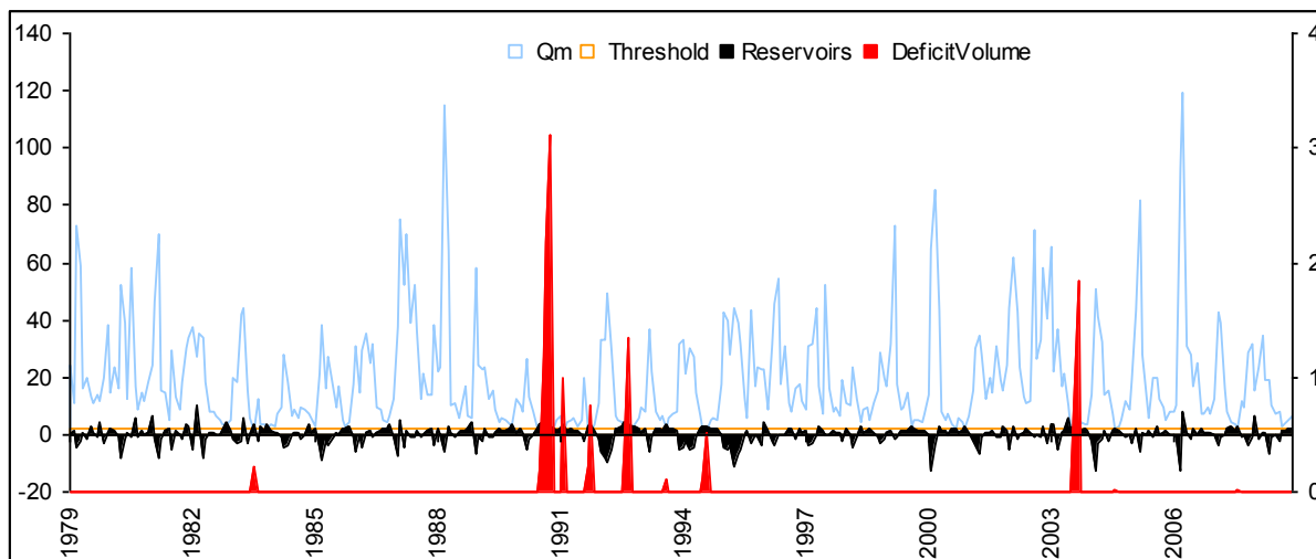
Obr. 8 Manipulace na kontrolním profilu Nespeky (černě) a deficitní objemy (červeně) pro threshold Q95%
