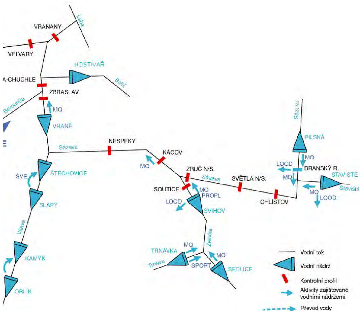
Obr. 6 Základní struktura vodohospodářské soustavy v dílčím povodí Dolní Vltavy
