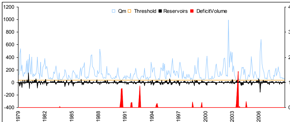
Obr. 9 Manipulace na kontrolním profilu Praha-Chuchle (černě) a deficitní objemy (červeně) pro threshold Q95%
