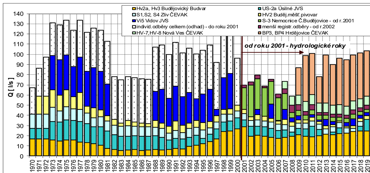
Obr. č. 12 Časový vývoj odběrů podzemní vody v průměrných ročních množstvích v hydrogeologickém rajonu 2160 v období kalendářních roků 1970-2019 (v l/s)
