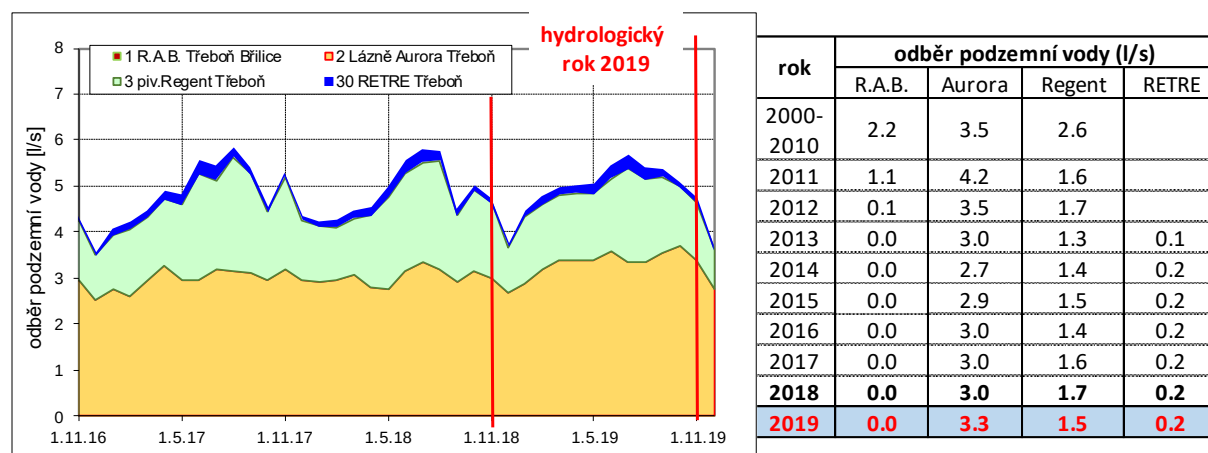
Obr. č. 7 Celkové odběry podzemní vody v lokalitě Třeboň v hydrologických letech 2000-2019 (v l/s)
