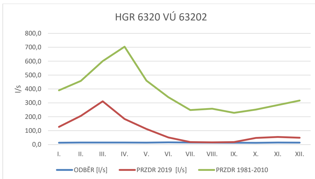
Graf č. 3 Zobrazení velikosti odběrů podzemní vody a přírodních zdrojů 2019 (PRZDR 2019) a přírodních zdrojů 1981-2010 (PRZDR 1981-2010) v HGR 6320 vodního útvaru 63202 v jednotlivých měsících
