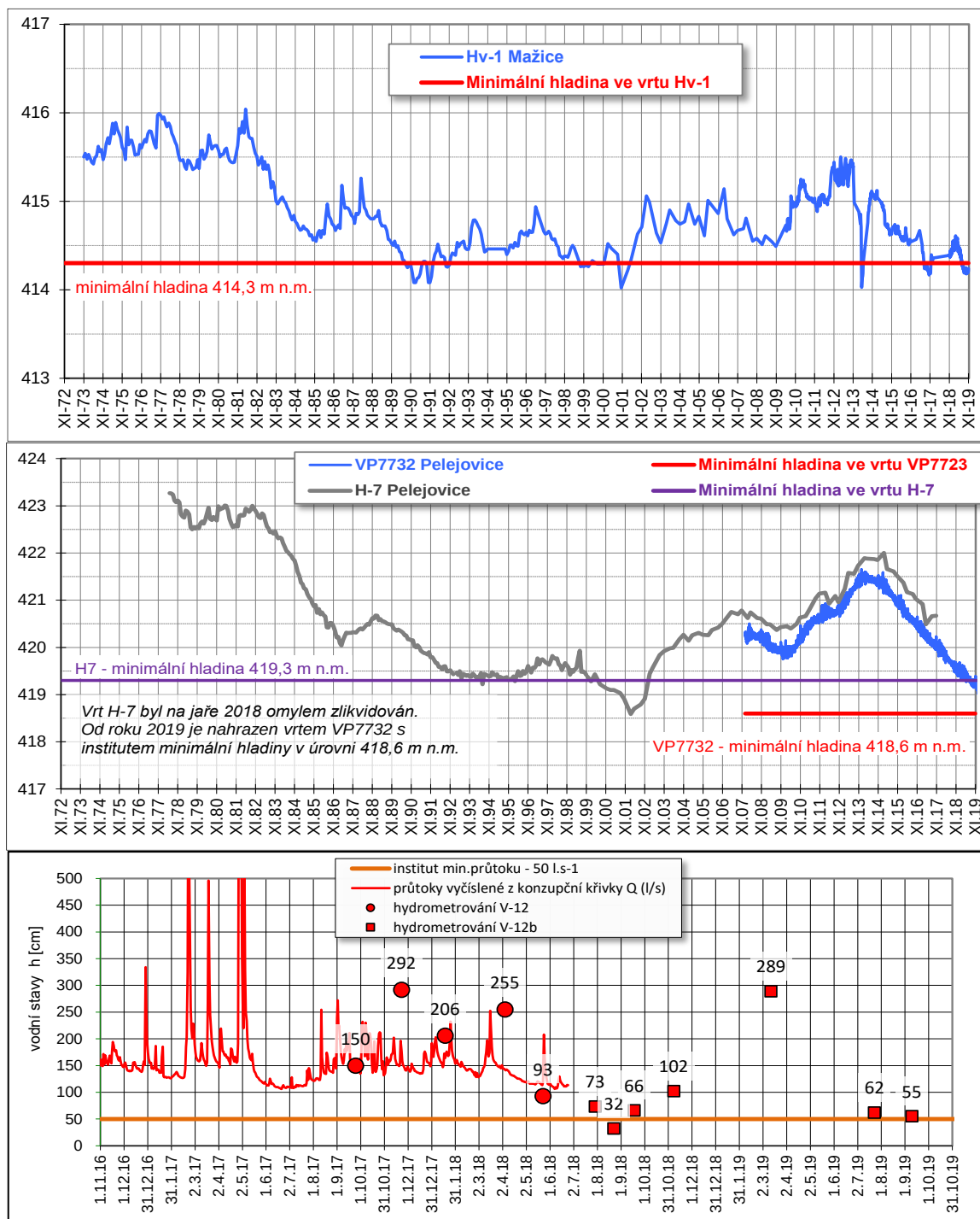
Obr. č. 10 Horusická jímací linie - uplatnění institutu minimální hladiny a úrovně hladin registrované v rámci režimního měření hladin podzemní vody ve vrtech HV1 Mažice a VP 7723 (pův. H7) Pelejovice v letech 1972-2019 a úroveň základního odtoku na Bechyňském potoce v profilu V-12 (V 12 b) Veselí n. L. (v letech 1981-2019)
