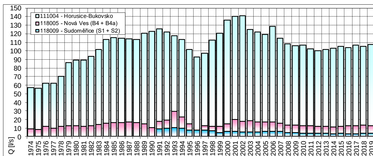
Obr. č. 8 Časový vývoj nejvýznamnějších odběrů podzemní vody v HGR 2151 (roční průměry 1974-2019 v l/s)
