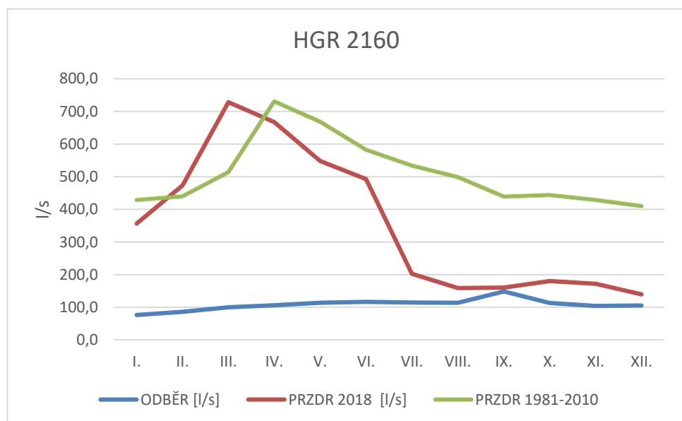
Graf č. 2 Zobrazení velikosti odběrů podzemní vody a přírodních zdrojů 2019 (PRZDR 2019) a přírodních zdrojů 1981-2010 (PRZDR 1981-2010) v HGR 2160 v jednotlivých měsících
