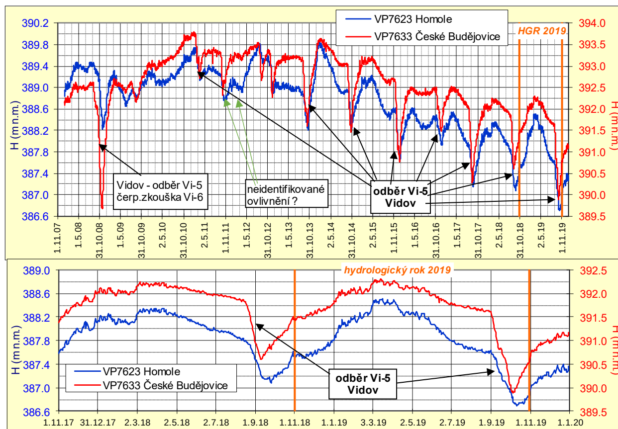
Obr. č. 13 Hladiny podzemní vody ve vrtech státní monitorovací sítě ČHMÚ v jižní části pánve (hlubší horizont - v m n.m.)
