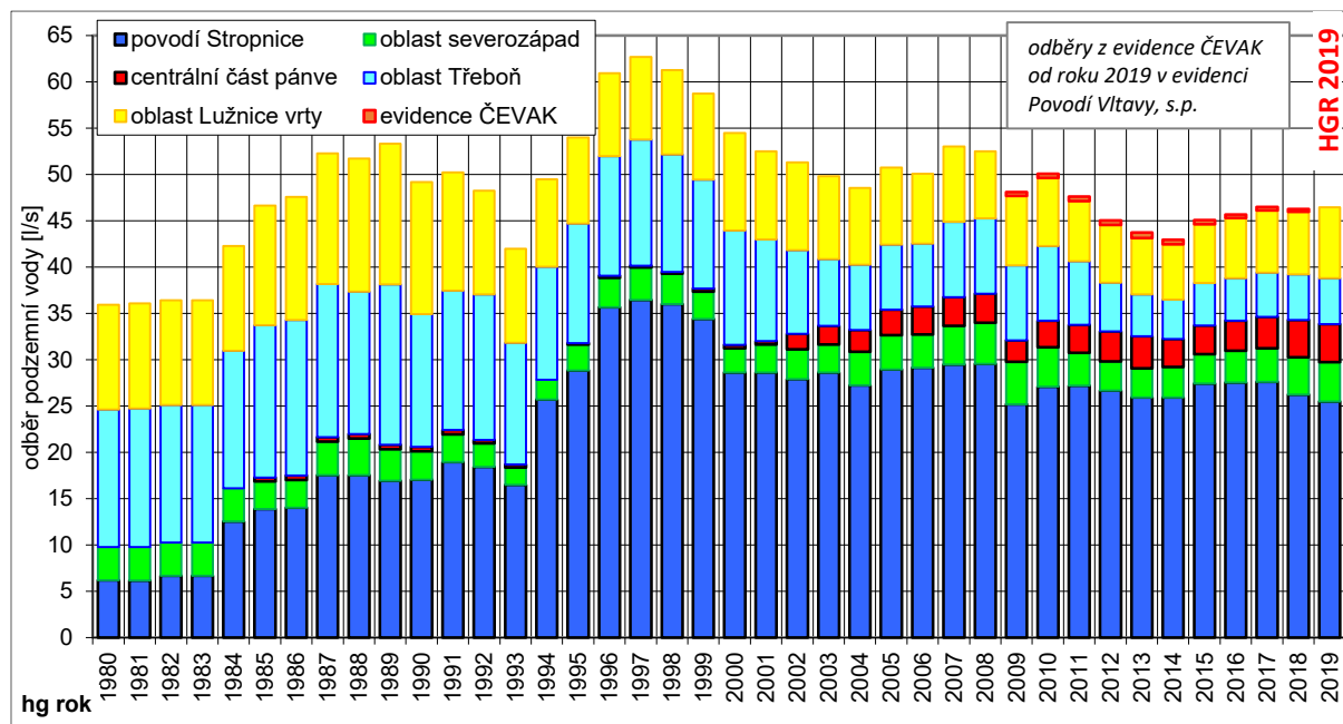
Obr. č. 3 Vývoj odběrů podzemních vod v nejvýznamnějších jímacích oblastech HGR 2140 v letech 1980-2019 (v l/s)
