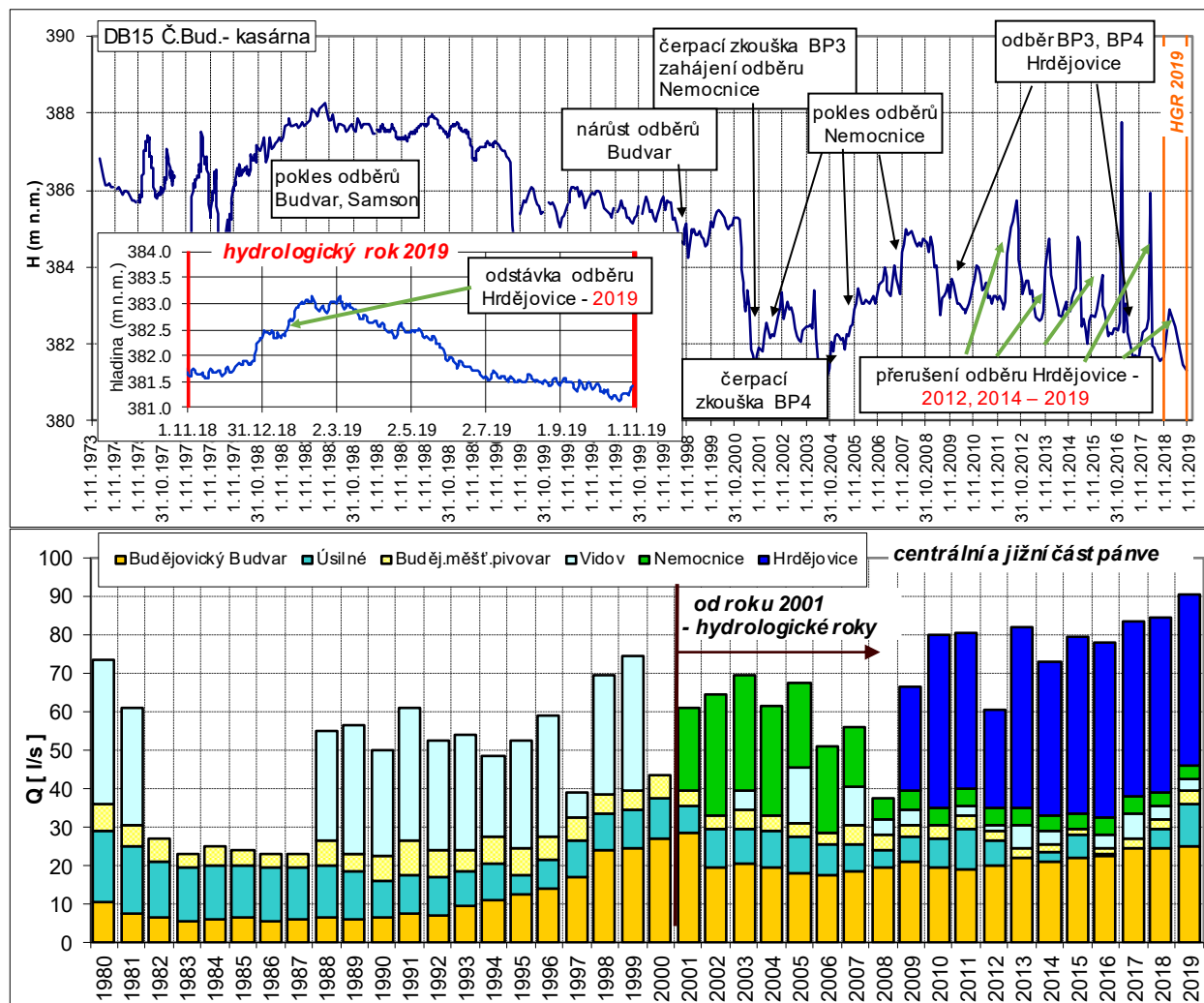
Obr. č. 15 Porovnání časového průběhu hladin podzemních vod (m n.m.) ve vrtu DB15 kasárna – Čtyři Dvory (1973-2019) s časovým vývojem vybraných odběrů podzemní vody v centrální a jižní části HGR 2160 v období hydrologických roků 1980-2019 (v l/s)
