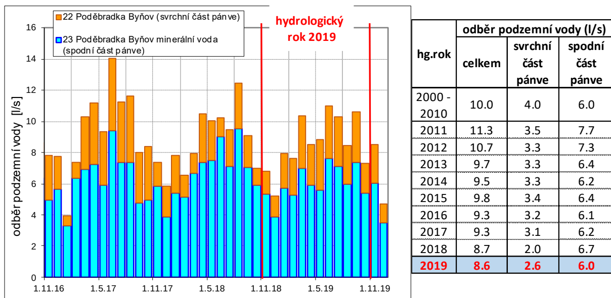
Obr. č. 4 Celkový odběr podzemní a minerální vody společnosti Poděbradka Byňov a.s. v lokalitě Tomkův mlýn v hydrologických letech 2000-2019 (v l/s)
