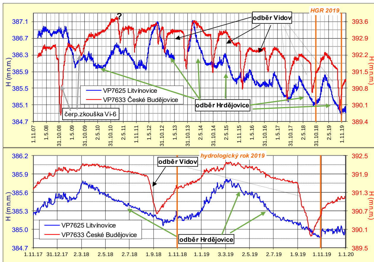
Obr. č. 14 Hladiny podzemní vody v centrální a jihozápadní části HGR 2160 ve vrtech státní monitorovací sítě ČHMÚ (hlubší části pánve – v m n. m.)
