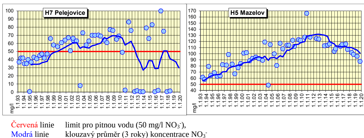
Obr. č. 20 Koncentrace dusičnanů v podzemní vodě v oblasti jižně od jímací linie Horusice-Dolní Bukovsko
