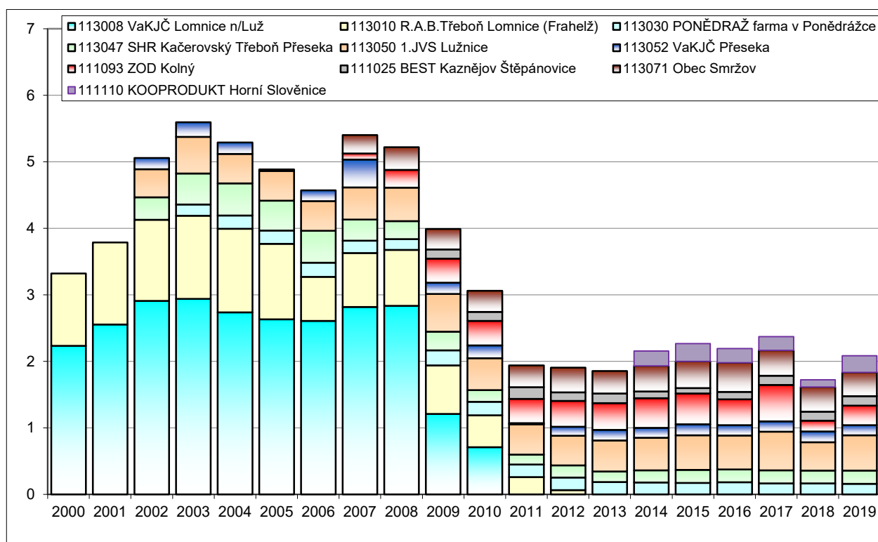
Obr. č. 11 Časový vývoj odběrů podzemní vody v hydrogeologickém rajonu 2152 v letech 2000-2019 (v l/s)
