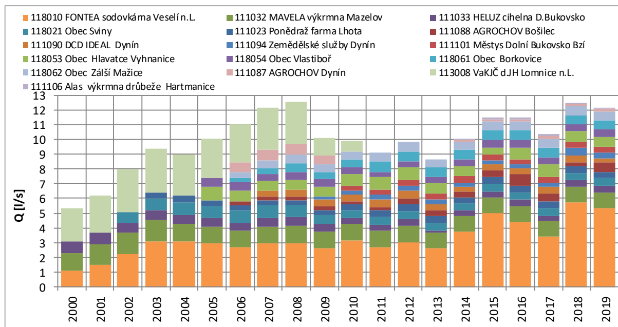
Obr. č. 9 Časový vývoj ostatních odběrů podzemní vody v HGR 2151 (roční průměry 2000-2019 v l/s)
