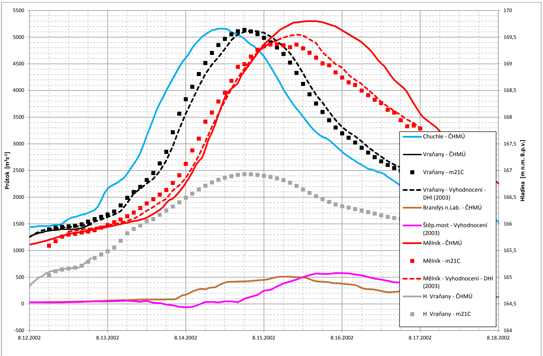
Příloha 3 – Rekonstrukce povodňové vlny 8/2002, výsledek simulace - model „Klecany – Mělník“
