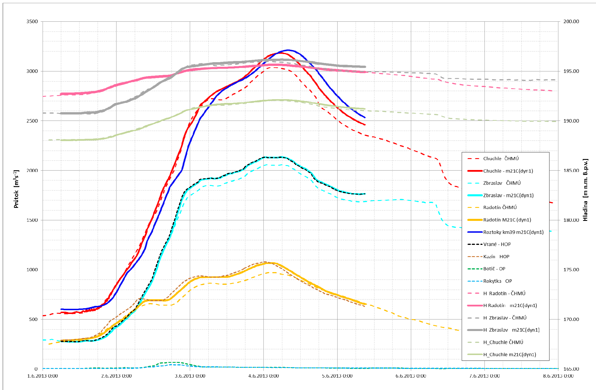
Příloha 1 – Rekonstrukce povodňové vlny 6/2013, výsledek simulace - model „Praha“
