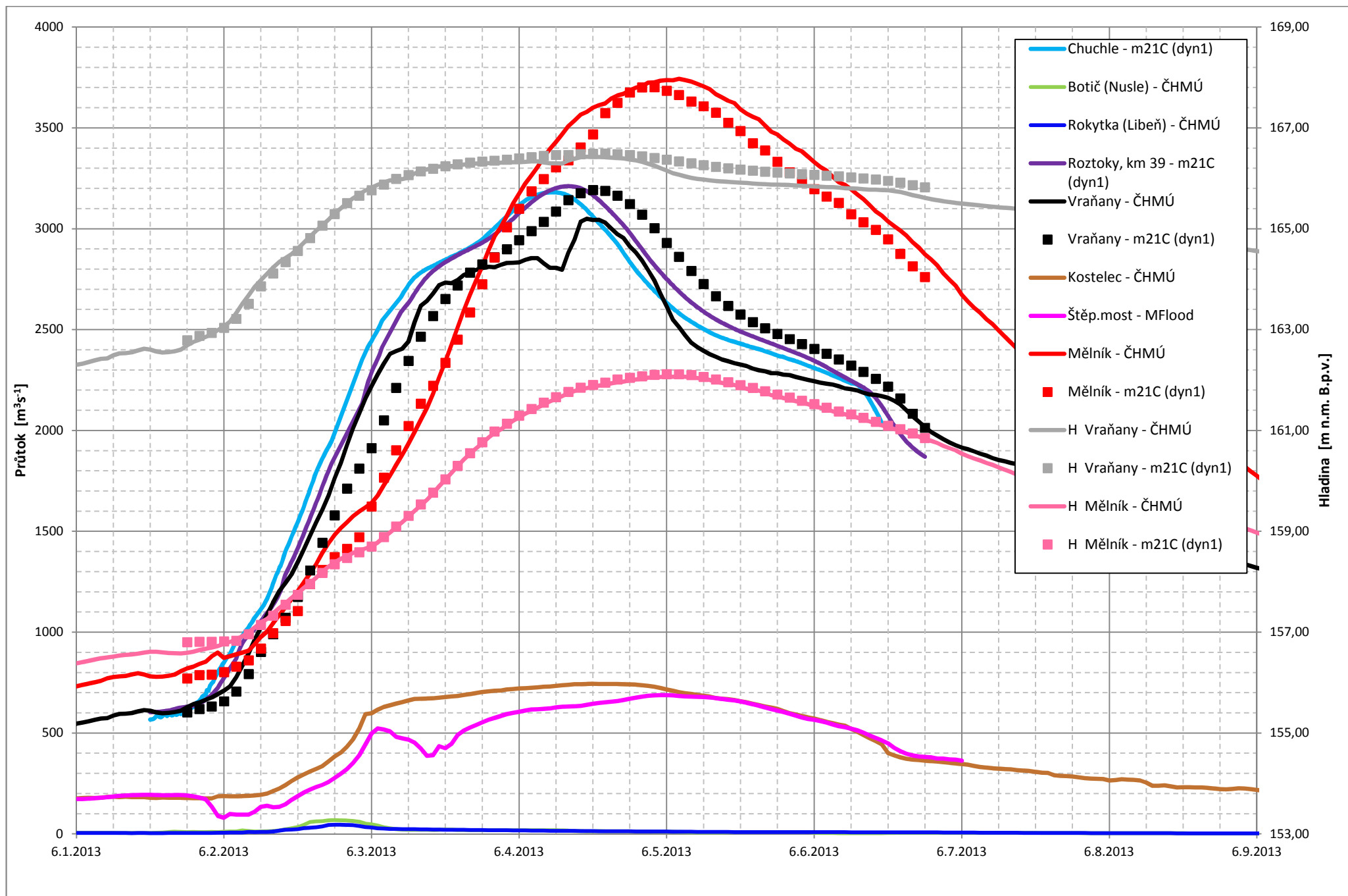
Příloha 2 – Rekonstrukce povodňové vlny 6/2013, výsledek simulace - model „Klecany – Mělník“
