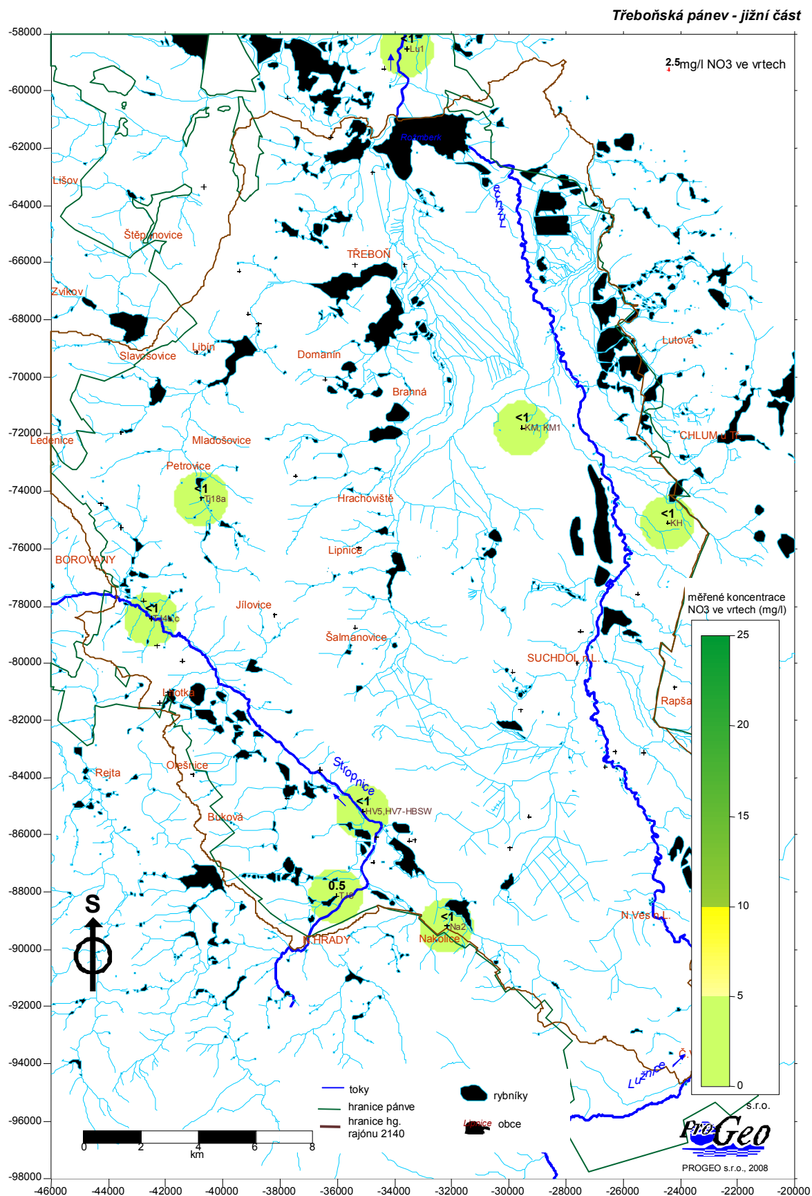
Obr. č. 22 HGR 2140 Situace s distribucí \text{NO}_3^- v podzemních vodách ve spodní části pánve
