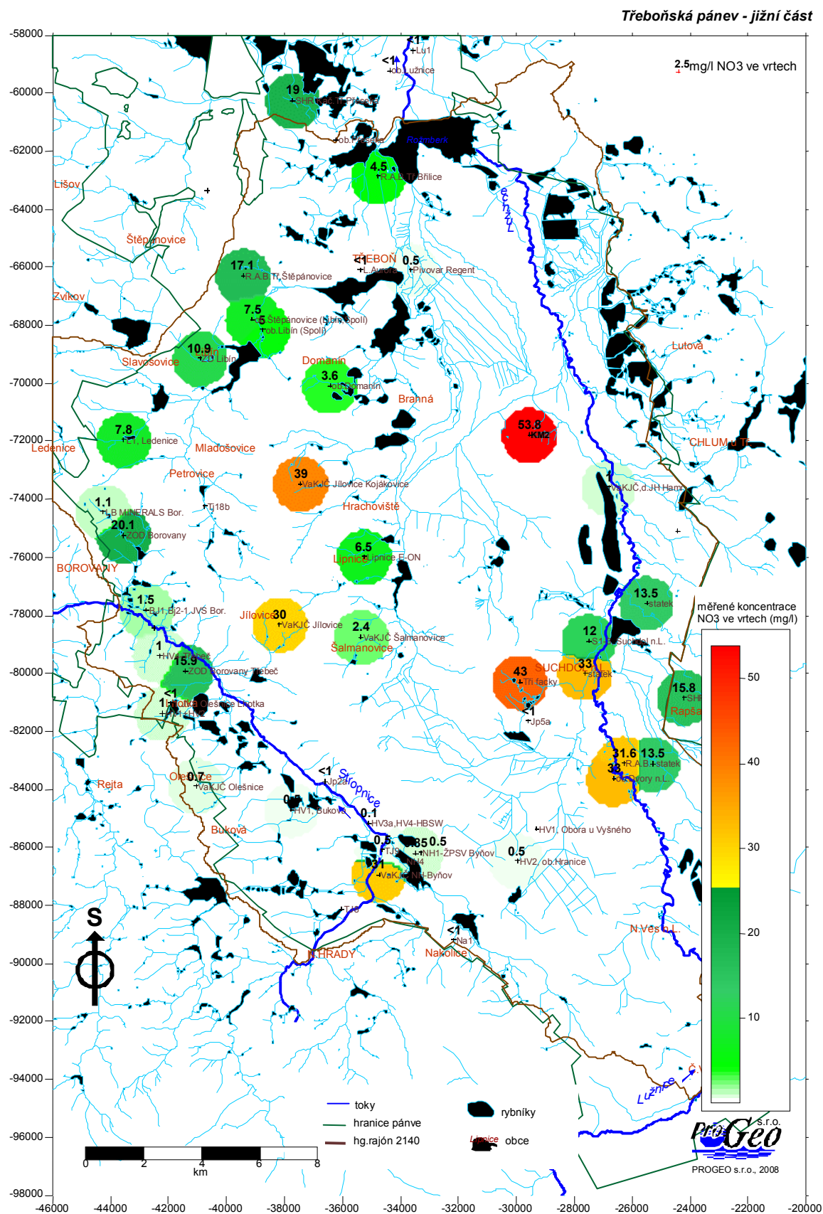
Obr. č. 21 HGR 2140 Situace s distribucí \text{NO}_3^- v podzemních vodách ve svrchní části pánve
