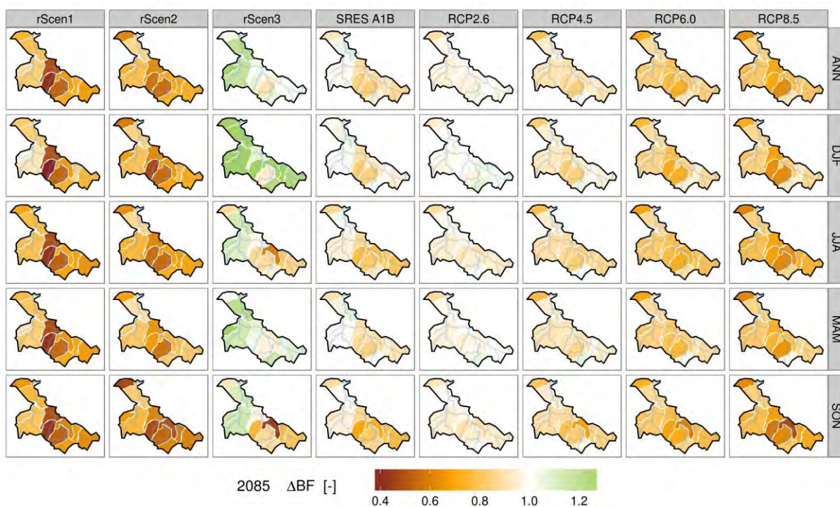
Obr. II.2.5c - Změna průměrných ročních výšek základního odtoku scénáře pro dílčí povodí Dolní Vltavy a rok 2085
