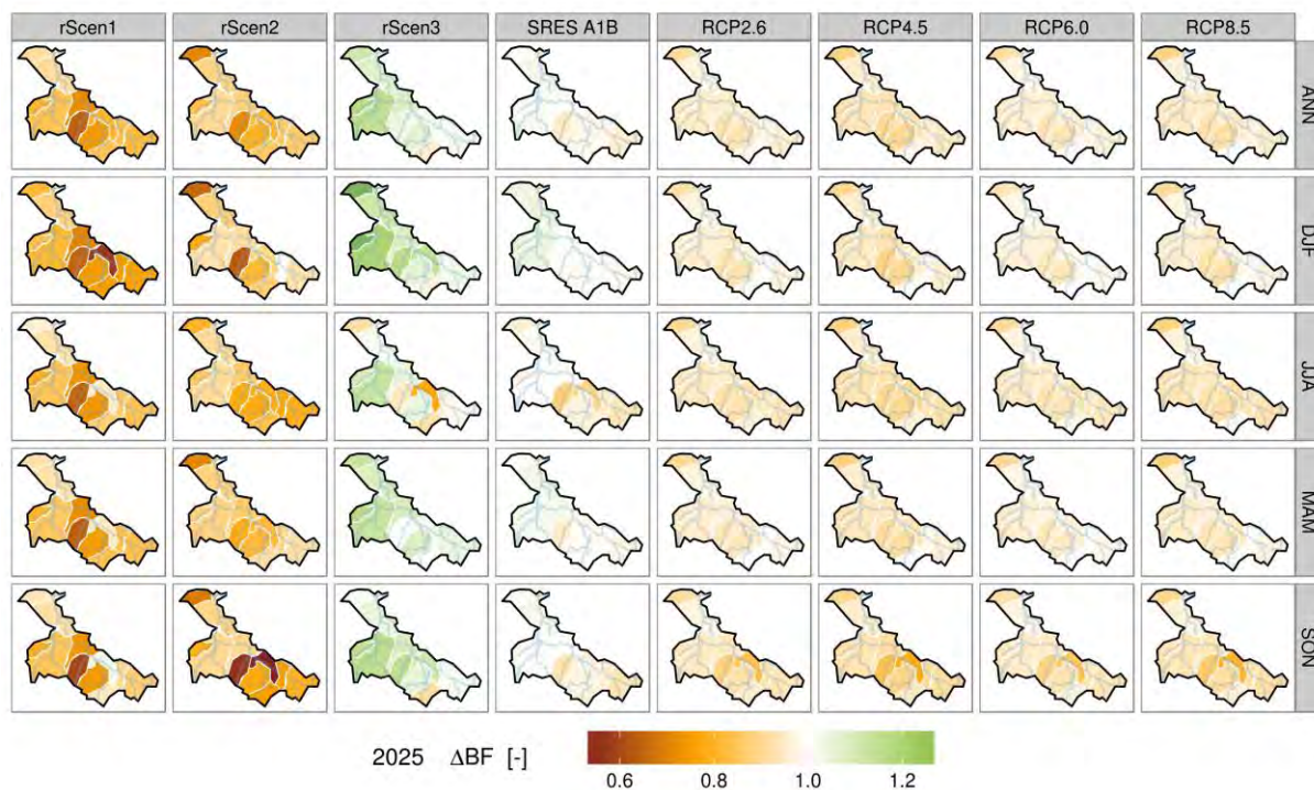
Obr. II.2.5a - Změna průměrných ročních výšek základního odtoku scénáře pro dílčí povodí Dolní Vltavy a rok 2025
