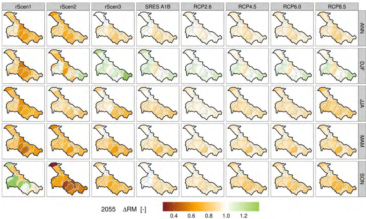
Obr. II.1.5h - Změna průměrných ročních odtokových výšek scénáře pro dílčí povodí Dolní Vltavy a rok 2055
