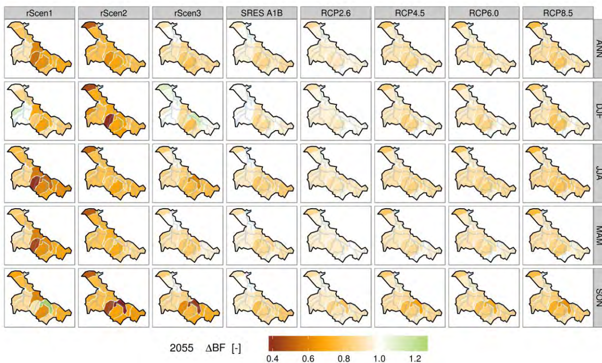
Obr. II.2.5b - Změna průměrných ročních výšek základního odtoku scénáře pro dílčí povodí Dolní Vltavy a rok 2055
