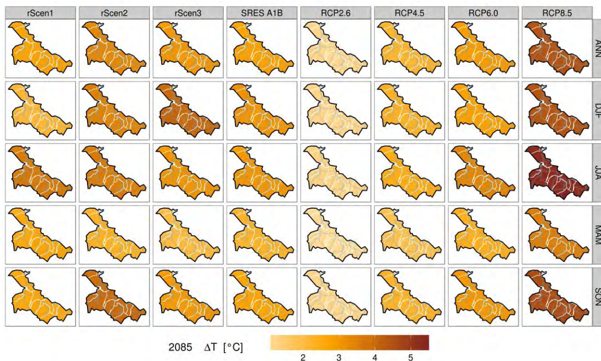
Obr. II.1.5f - Změna teploty pro dílčí povodí Dolní Vltavy a rok 2085
