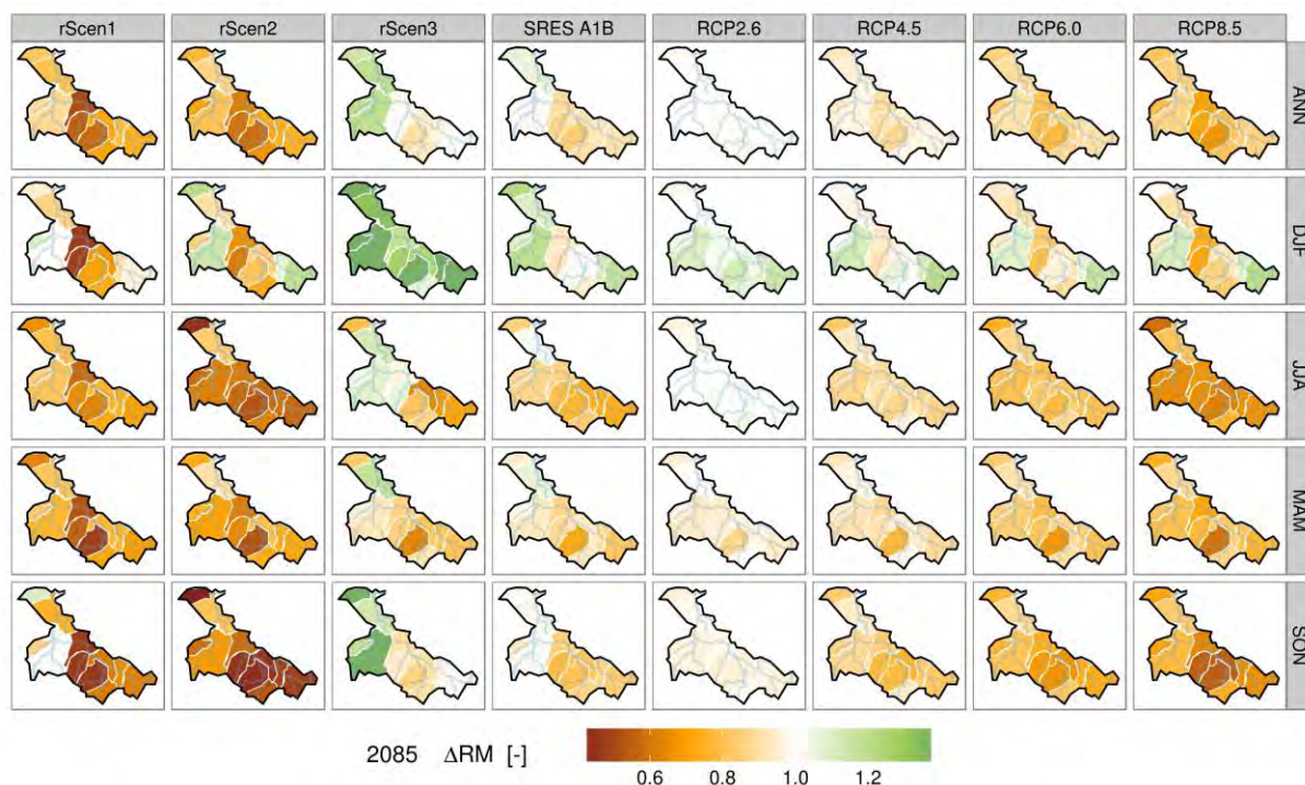
Obr. II.1.5i - Změna průměrných ročních odtokových výšek pro dílčí povodí Dolní Vltavy a rok 2085
