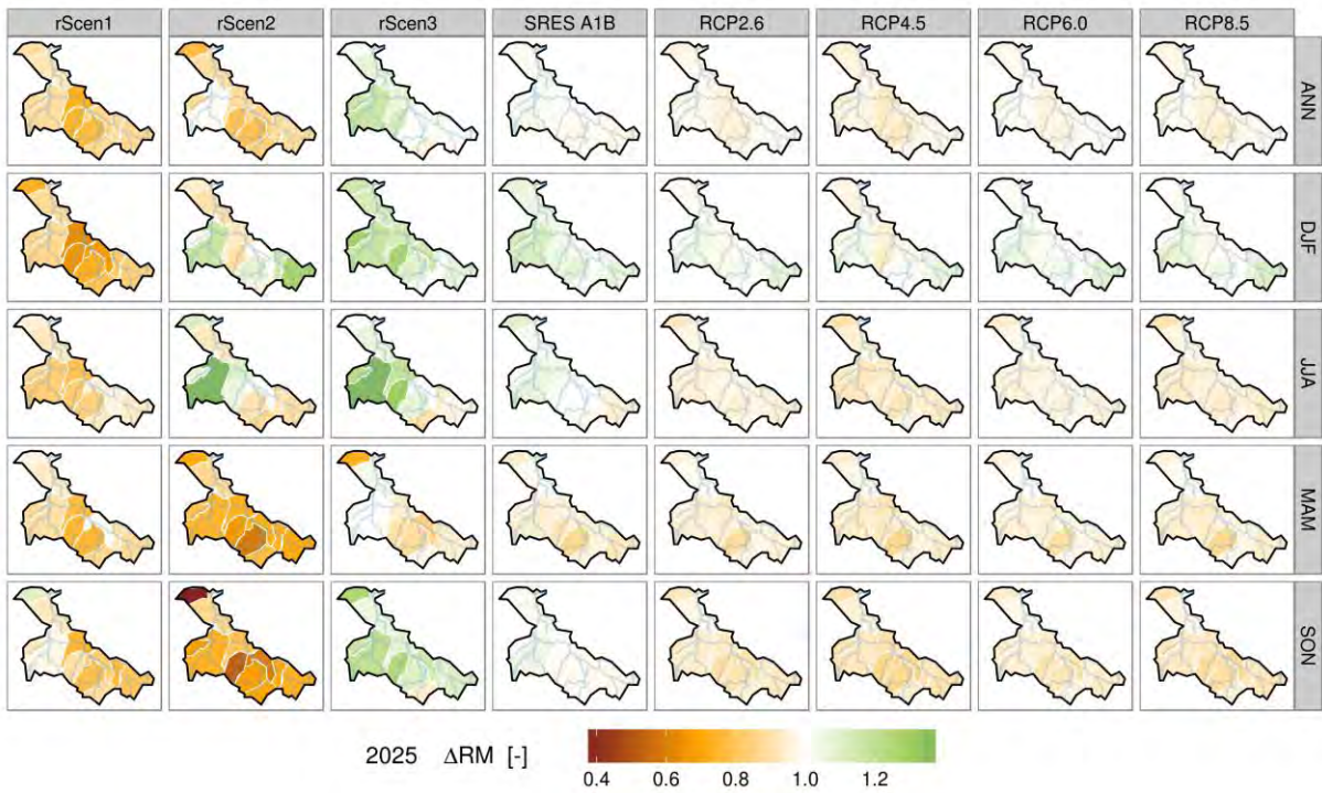
Obr. II.1.5g - Změna průměrných ročních odtokových výšek scénáře pro dílčí povodí Dolní Vltavy a rok 2025
