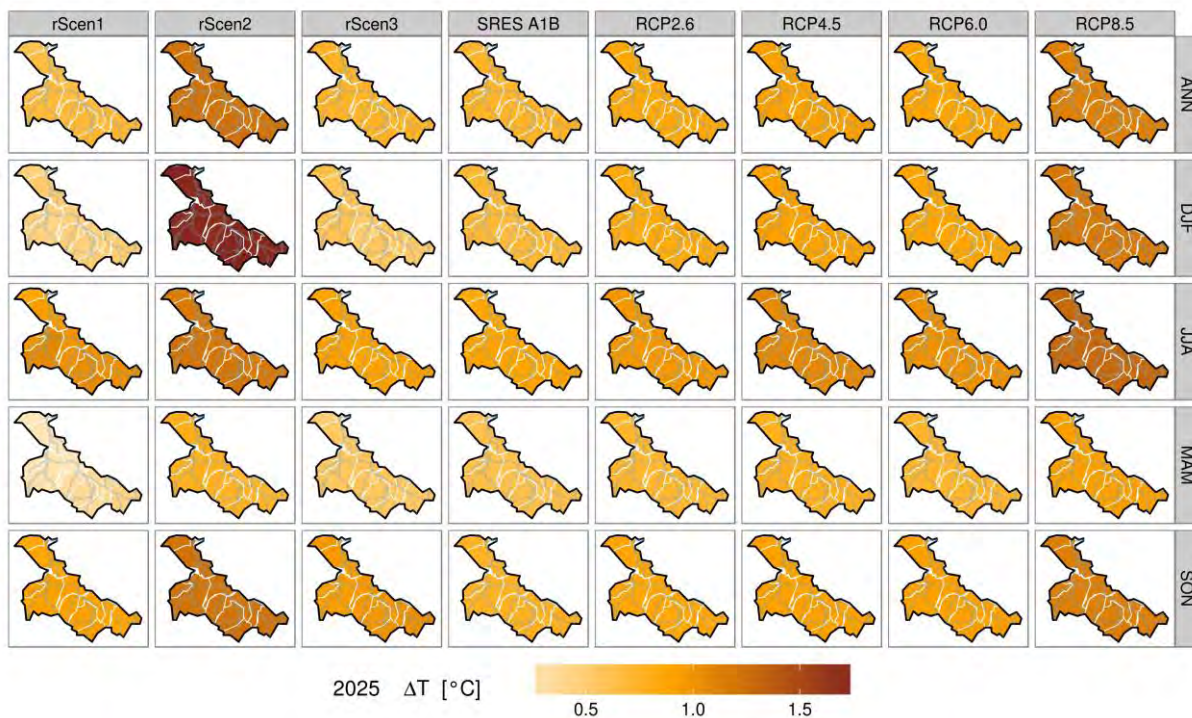
Obr. II.1.5d - Změna teploty pro dílčí povodí Dolní Vltavy a rok 2025
