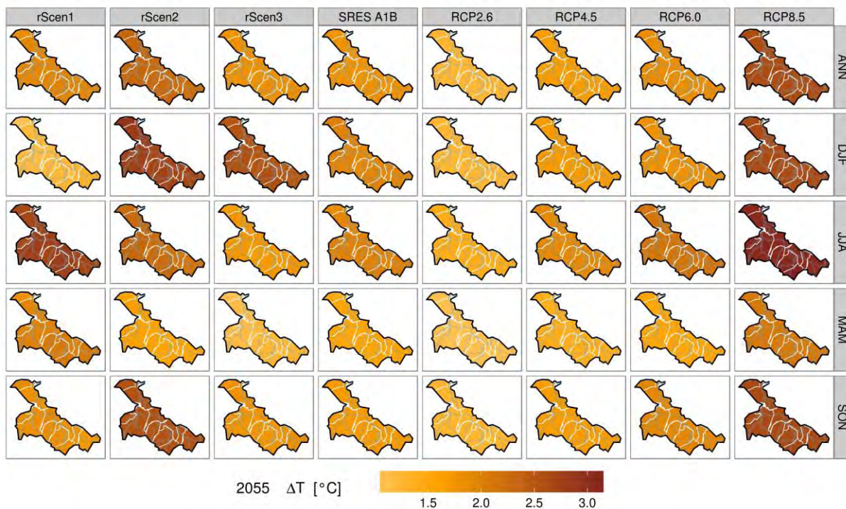
Obr. II.1.5e - Změna teploty pro dílčí povodí Dolní Vltavy a rok 2055
